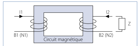
39 Le principe du TC utilisé en alternatif
