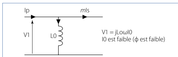
14 Le schéma équivalent en cas d'ouverture du secondaire du TC
